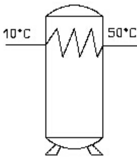
Abb. 2: Prinzipskizze für einen Speicher mit starker Durchmischung
