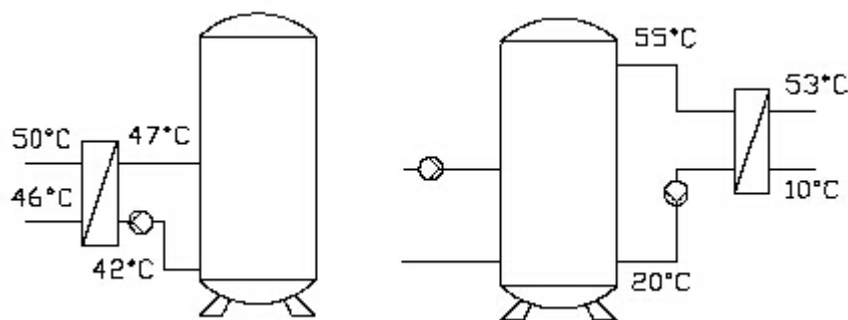
Abb. 3: Prinzipskizze für Speicherkonzepte mit externen Wärmetauschern
